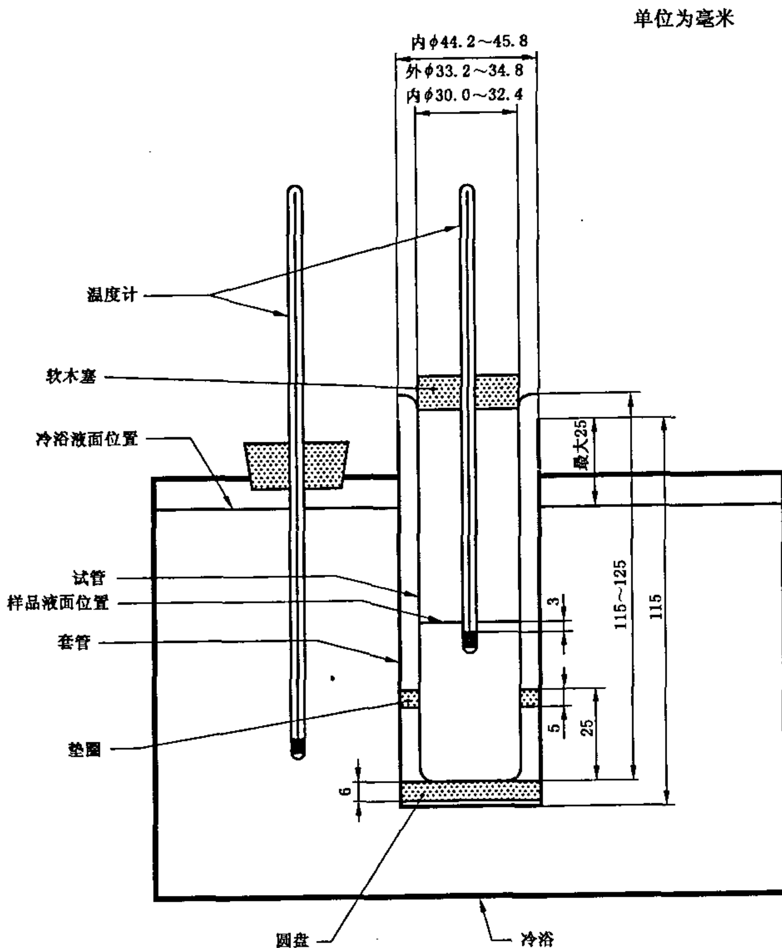
图1 倾点测定仪
