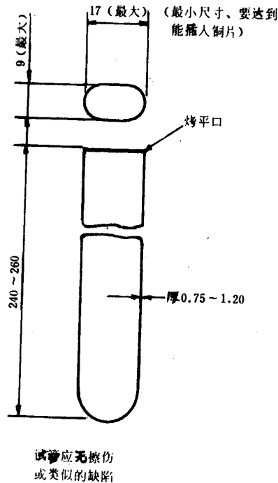
图 2 观察试管
