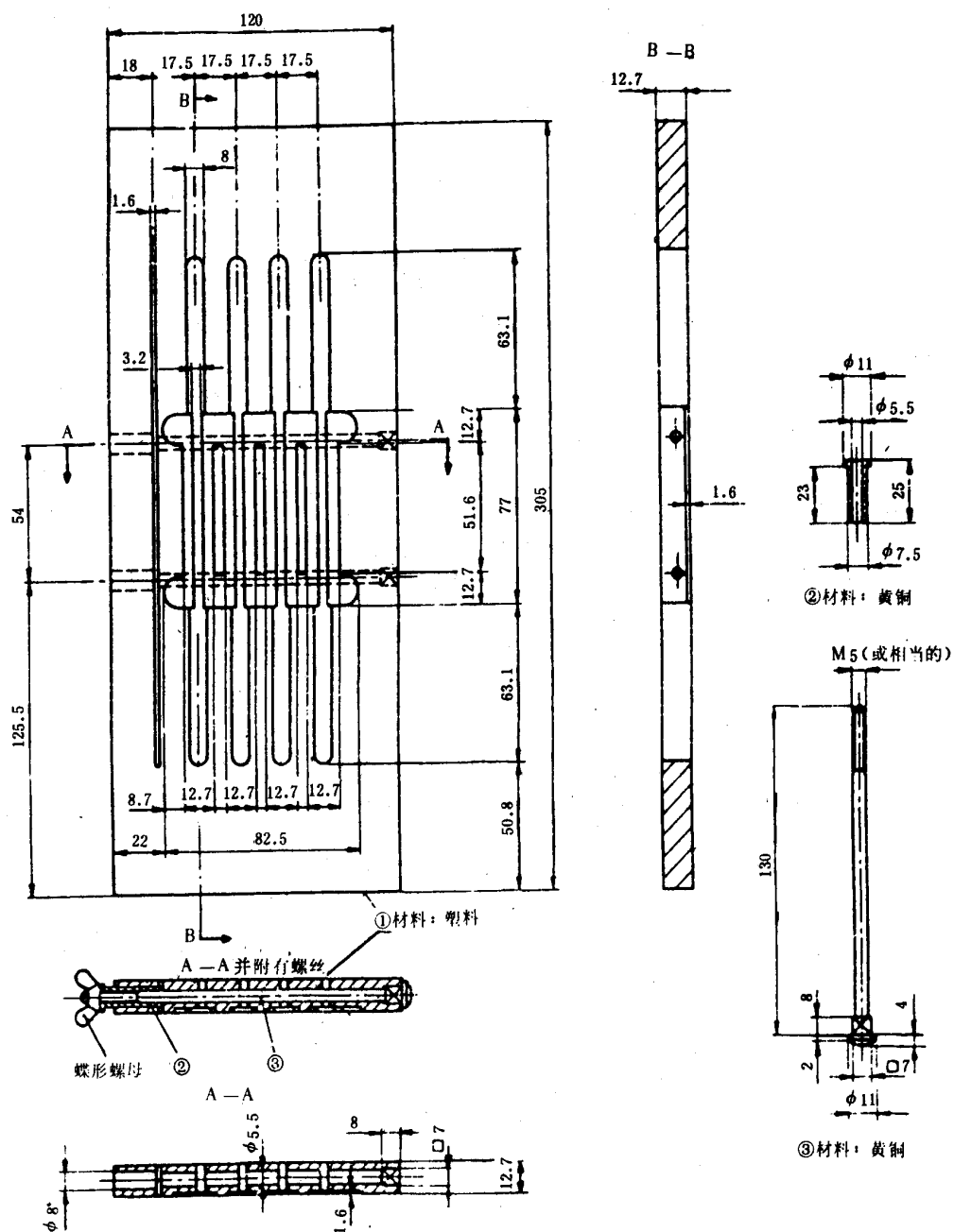
图 1 磨片夹具
