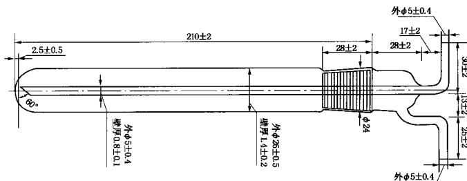
氧化管图
